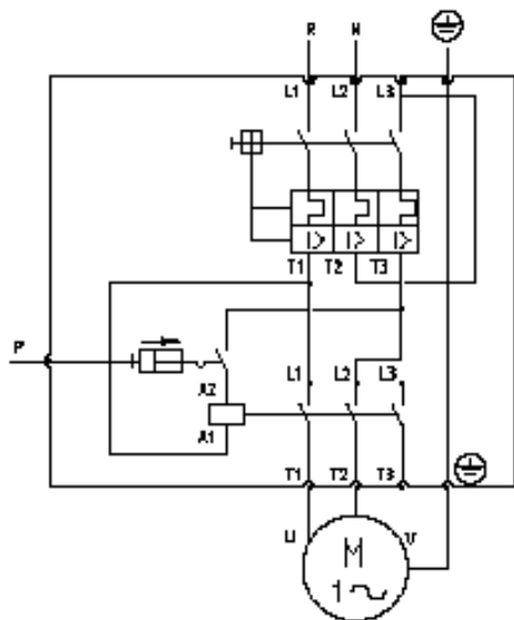
Однофазная сеть
