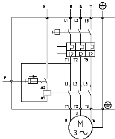
Трехфазная сеть
