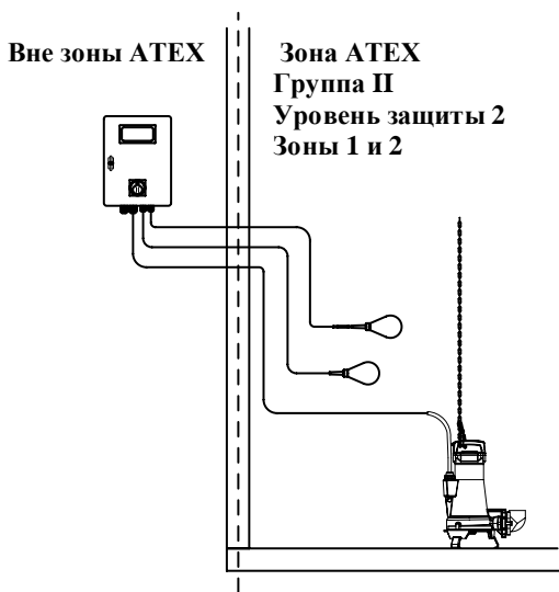
Рис. 3.1. Монтаж электрощита вне зоны АТЕХ
