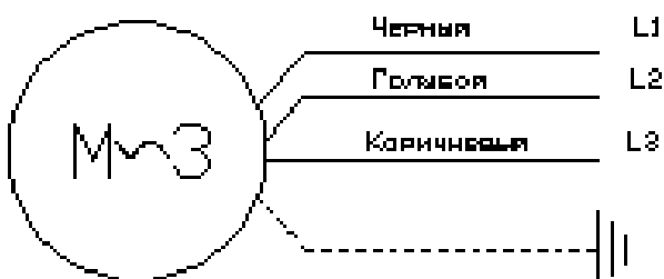
Схема подключения трехфазного насоса
