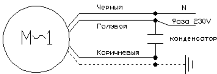
Схема подключения однофазного насоса
